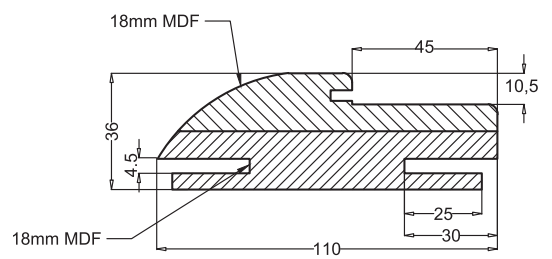
36x110x2100 BOMBELİ KASA
